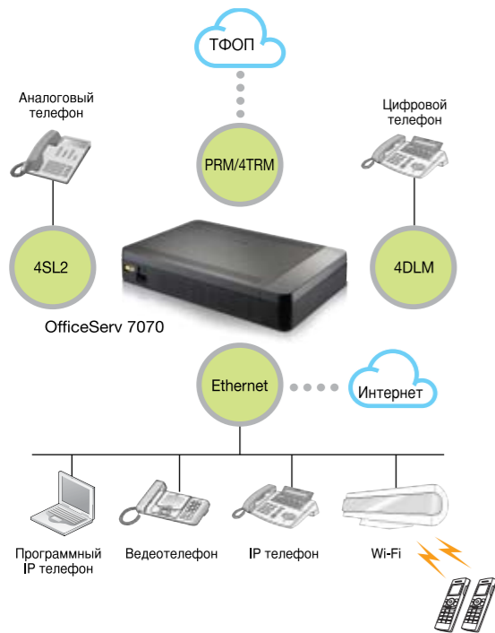
Конфигурация линий системы OfficeServ 7070
